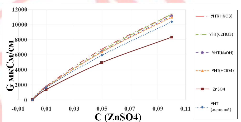
Рис. 1. Зависимость электропроводности растворов сульфата цинка от модифицированных МУНТ.
