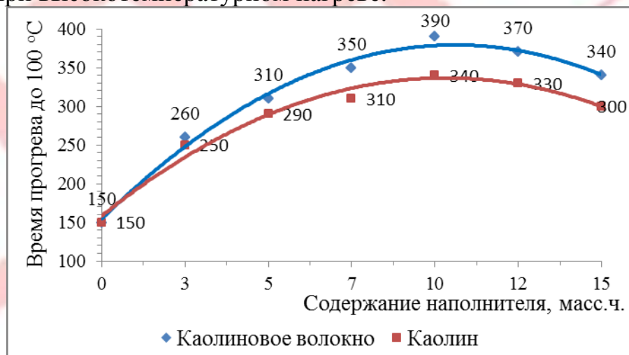
Рис. 1. Зависимость времени прогрева до 100 °C от содержания наполнителя.
