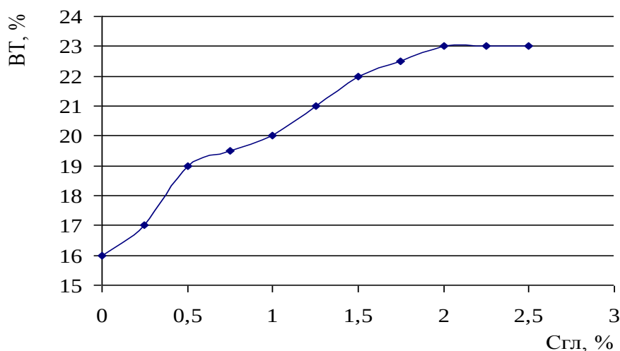
Рис. 1. Влияние концентрации глицерина на выход по току хрома. Катод - графит; анод - свинец (2 шт); V=200 мл; \text{CrO}_3 =50 г/л; \text{H}_2\text{SO}_4 =2,5 г/л; D_k =10 А/дм 2 ; t=50-60° С.
