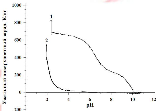
Рис. 1 График зависимости удельного поверхностного заряда от pH: 1 – немодифицированный ZrO_2 ; 2 – модифицированный ZrO_2 .
