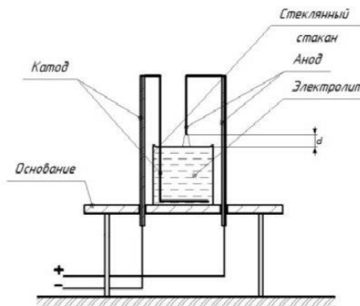
Рис. 1. Схематическое изображение рабочей камеры экспериментальной установки.
