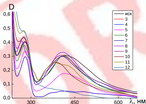
Рис.1. Спектры поглощения синтезированного нанокompозита при различных pH среды.
