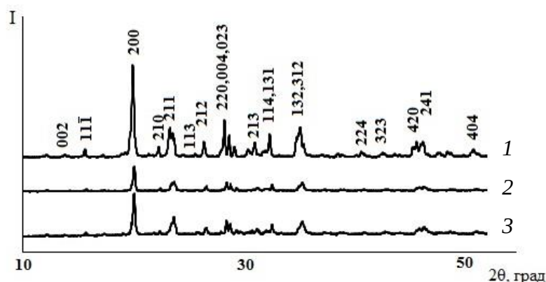
Рис. 1. Рентгенограммы фосфатов \text{Zn}_{0.5(1+x)}\text{Fe}_x\text{Zr}_{2-x}(\text{PO}_4)_3 : x = 0(1), 0.3(2), 0.4(3) .
