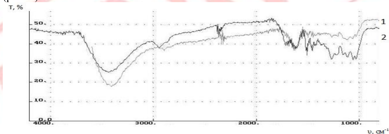
Рис. 1. ИК-спектры лигнина, модифицированного салициловой кислотой (1), и сульфатного лигнина (2).
