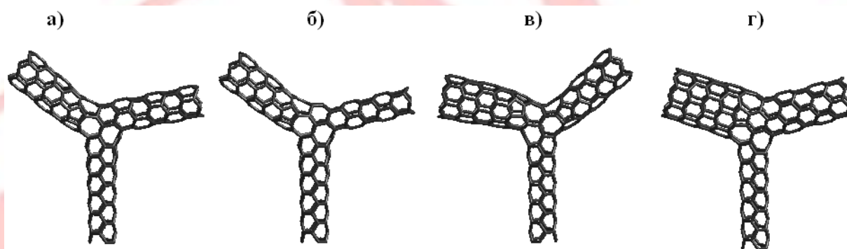
Рис. 1. Y-образные гетероструктуры на основе углеродных нанотрубок: а) УНТ (6,0) – (5,0) – (3,3); б) УНТ (6,0) – (4,0) – (3,3); в) УНТ (7,0) – (6,0) – (3,3); г) УНТ (8,0) – (6,0) – (3,3).
