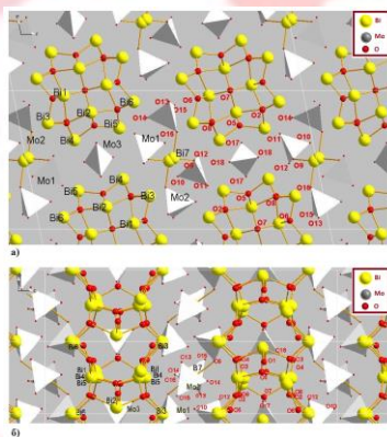
Рис.1. Структура \text{Bi}_{13}\text{Mo}_5\text{O}_{34\pm\delta} .
