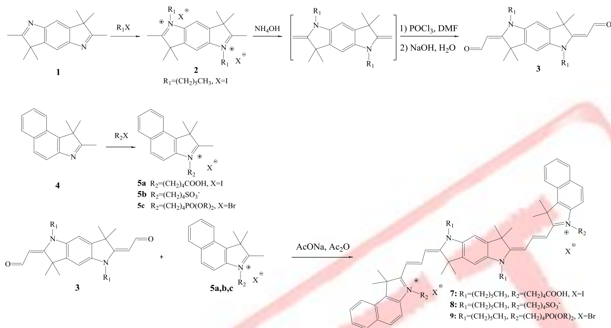
Рис. 1. Схема синтеза.
