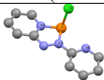
Рисунок 1. Молекулярная структура 5.
