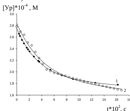
Рис. 1. Рассчитанная (1) и экспериментальная (2) кинетические кривые расщепления 5-гидрокси-6-метилурацила. [Ур]_0 = 2.8 \times 10^{-4} моль/л, V_i = 4 \times 10^{-7} 348 К.
