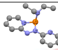
Рисунок 2. Молекулярная структура 4.
