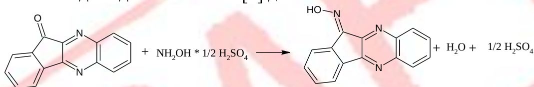
Рис. 1. Схема взаимодействия 11Н–индено[1,2-б]хиноксалинона с гидроксилaminом сернокислым.
