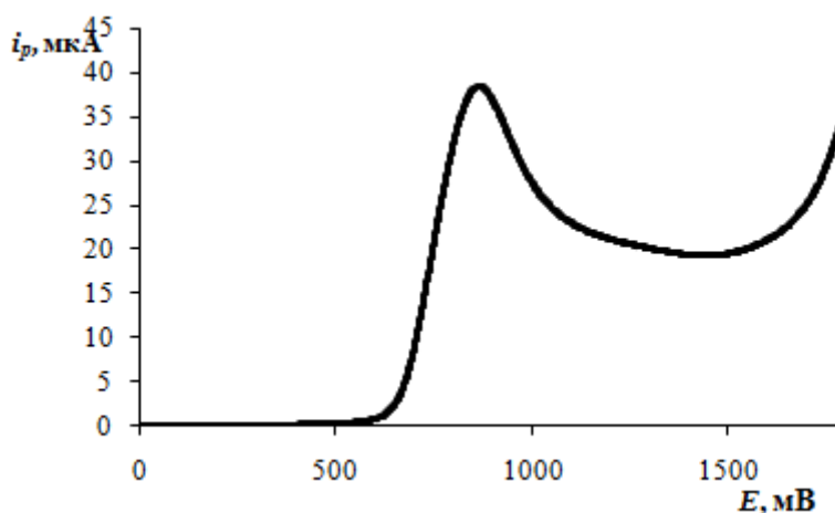
Рис.1. Линейная вольтамперограмма окисления 0,0245 мМ раствора триптофана на СУЭ, модифицированном полиариленфталидом SOO; на фоне фосфатного буферного раствора (pH 6,86), \nu = 0,1 \text{ В/с.} , t_{\text{н}} = 30 \text{ сек.}
