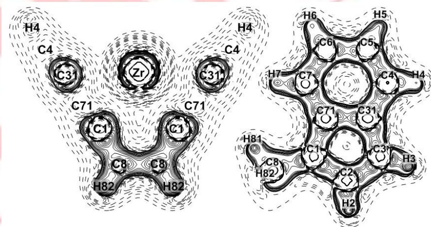
Рис. 1. Квантовая компонента распределения внутреннего электронного давления в цирконоцене рац-этилен-бис(1-инденил) цирконий дихлорид.
