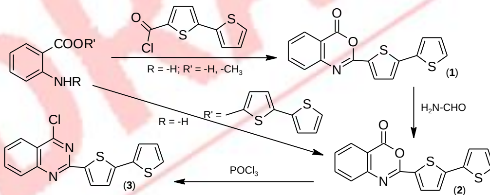
Рис. 1. Схема синтеза.
