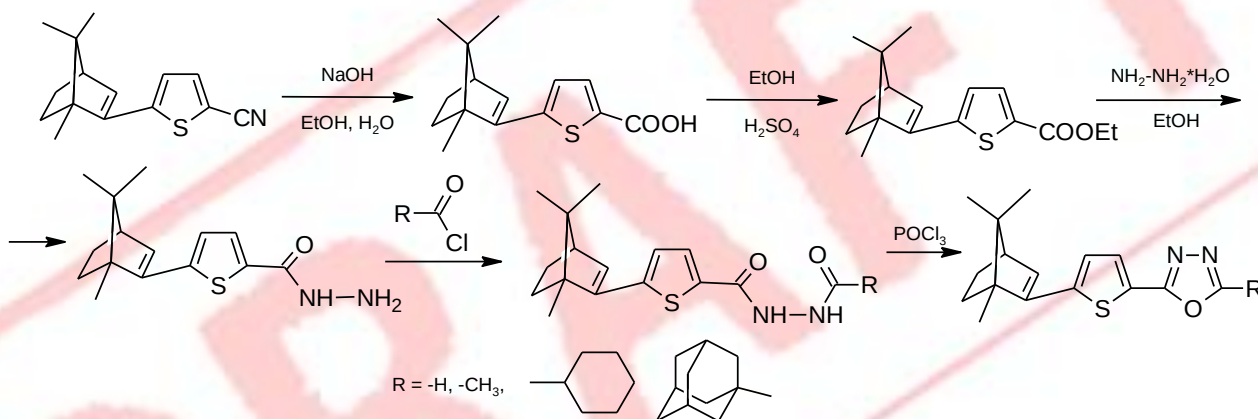
Рис. 1. Схема синтеза.
