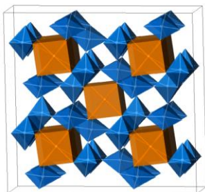
Рисунок 1. Фрагмент структуры \text{BaAl}_2\text{Ti}_6\text{O}_{16} , построенный на основе данных, полученных методом Ритвельда.
