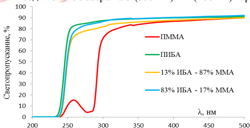
Рис. 1. Оптическая прозрачность сополимеров ИБА с ММА.
