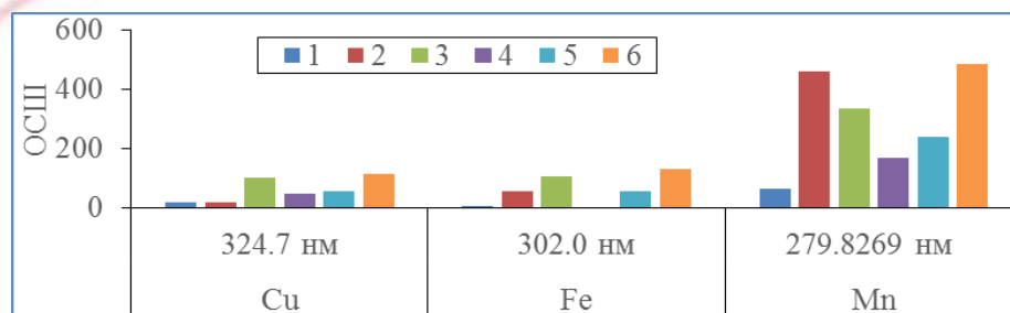
Рис.2. Отношение сигнал-шум(ОСШ) для различных видов электродов.
