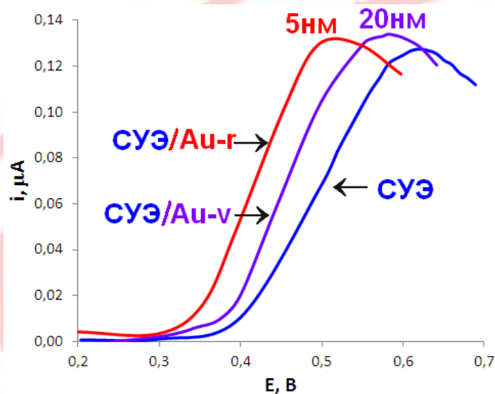
Рис. 1 Экспериментальные вольтамперограммы электроокисления 2 \times 10^{-5} М мочевины на немодифицированном СУЭ и СУЭ, модифицированном наночастицами золота
