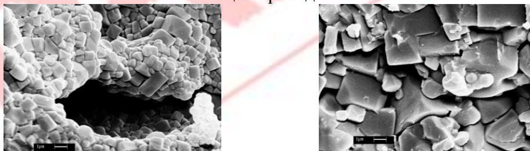
Рис. 1. SEM таблеток LATP после спекания при 1000°C в течение 1 ч и 6 ч.
