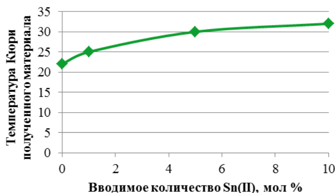
Рис. 1. Изменение температуры Кюри образцов SbSI, легированных катионами Sn(II).
