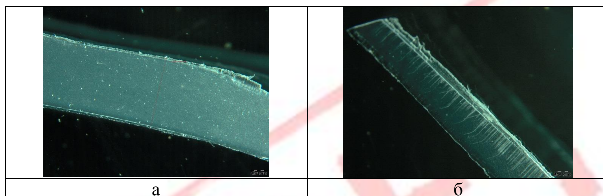
Рисунок 1. Микрофотография единичного волокна образца 1 (а) и 2 (б).
