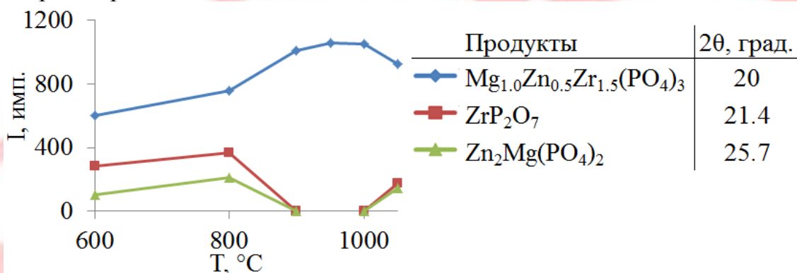
Рис. 1. Влияние температуры на формирование \text{Mg}_{1.0}\text{Zn}_{0.5}\text{Zr}_{1.5}(\text{PO}_4)_3 .
