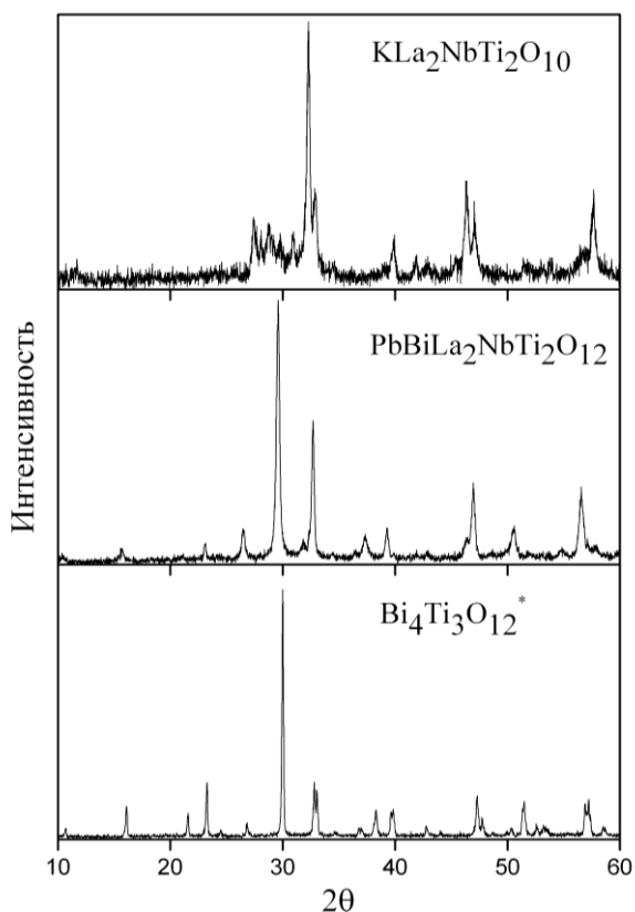
Рис. 1. Рентгенограммы соединений \text{KLa}_2\text{NbTi}_2\text{O}_{10} , \text{PbBiLa}_2\text{NbTi}_2\text{O}_{12} и \text{Bi}_4\text{Ti}_3\text{O}_{12}^* (* – типичный представитель фаз Ауривиллиуса)
