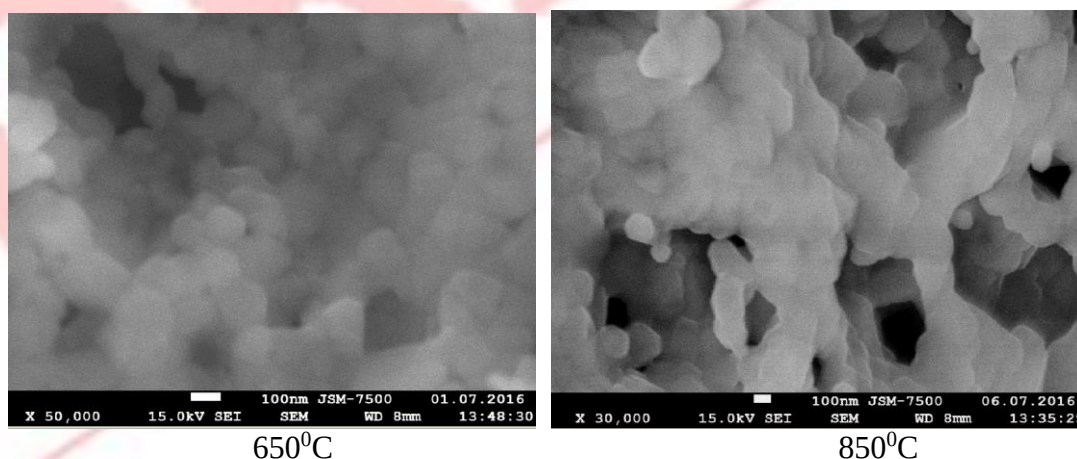
Рис. 1. Микрофотографии полученного пирохимическим нитрат-мочевинным методом LCZFO с 1 часовым отжигом при различных температурах
