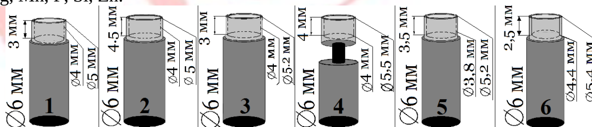
Рис.1. Параметры используемых электродов.
