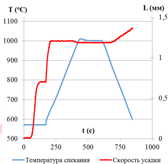
Рис. 1. Скорость усадки при получении керамического образца из наногидроксиапатита при 1000°C
