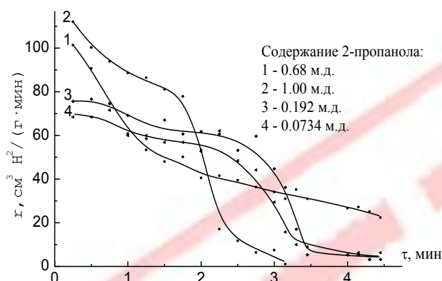
Рис. 1. Кинетические зависимости реакции гидрогенизации 4-нитрофенола на скелетном никеле в водных растворах 2-пропанола различных составов.
