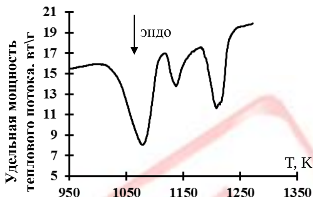
Рис 1. ДСК кривая соединения KNbTeO_6
