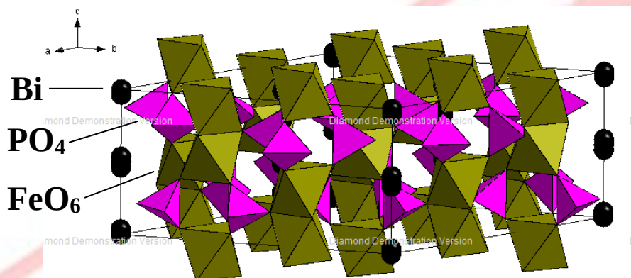
Рис. 1. Фрагмент структуры \text{BiFe}_2(\text{PO}_4)_3 .
