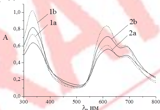
Рис. 1. ЭСП водных растворов композитов КМЦ с Со- фталоцианином (а- массовое содержание макроцикла в композите 1,1%; б – 1,2%) при ультразвуковом воздействии (1) и без него (2).
