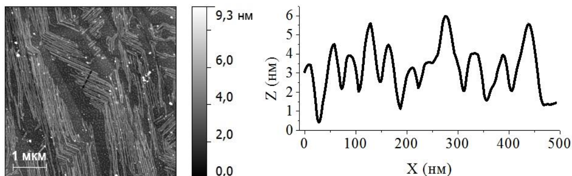
Рис. 1. АСМ изображение и профиль наноструктурированных полос кобальта на поверхности графита.
