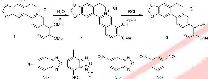
Рис. 1. Получение 9-нитроарилберберинов 3 .
