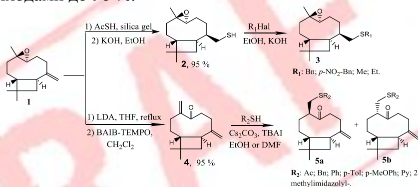
Рис. 1. Синтез тиопроизводных.
