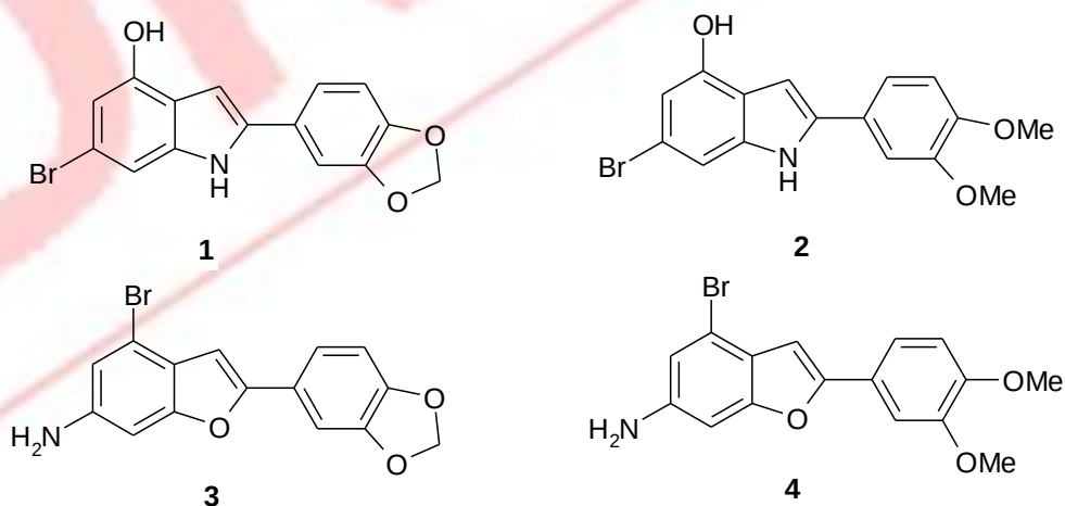
Рис. 1. Полученные соединения.
