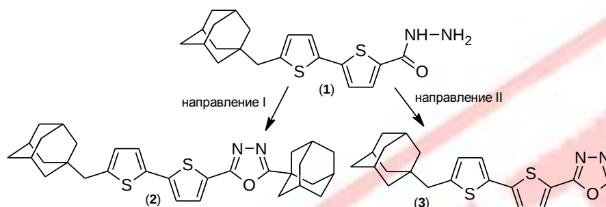
Рис. 1. Схема синтеза.
