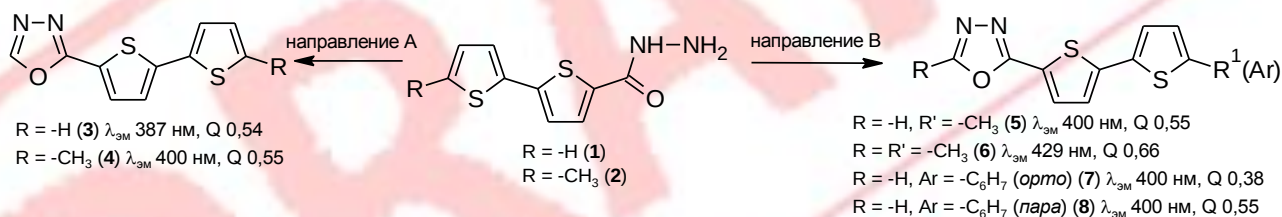
Рис. 1. Схема синтеза.
