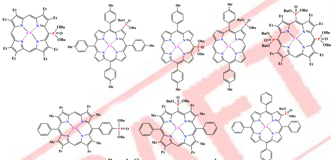
Рис. 1. Синтезированные порфирины.
