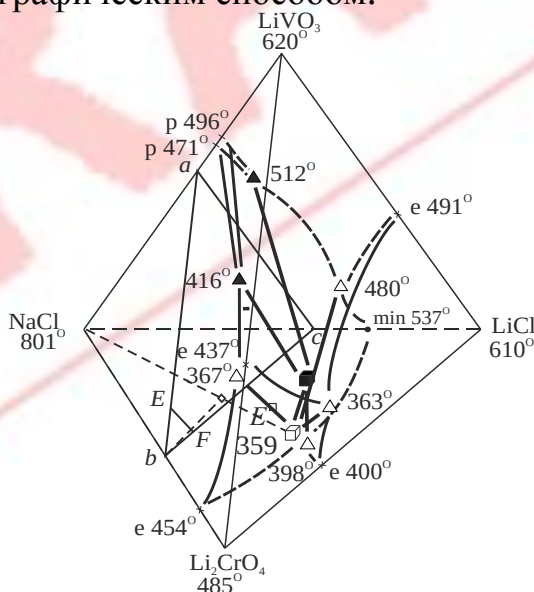
Рис. 1. Эскиз объемов кристаллизации стабильного тетраэдра \text{LiCl-LiVO}_3\text{-Li}_2\text{CrO}_4\text{-NaCl} .
