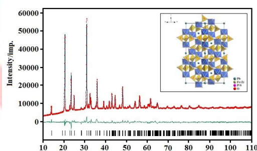
Рис. 3. Рентгенограмма \text{Pb}_{2/3}\text{FeZr}(\text{PO}_4)_{7/3}(\text{SO}_4)_{2/3}
