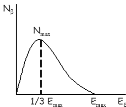
Рис. 1. Спектр \beta -частиц.
